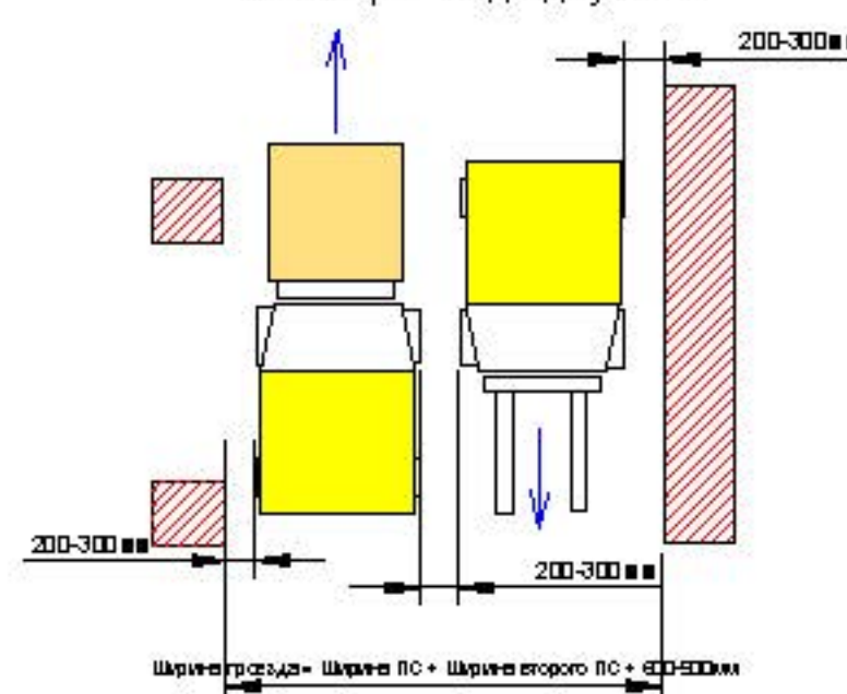
Схема разъезда двух ПС
